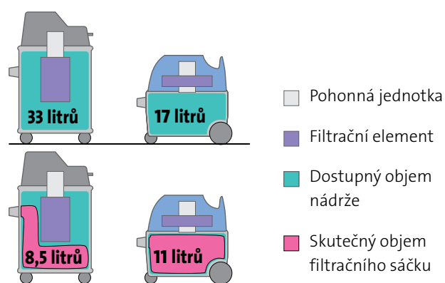
Běžný průmyslový vysavač Ventos 20 E/L
